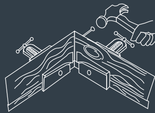
Ensamble de 2 piezas
