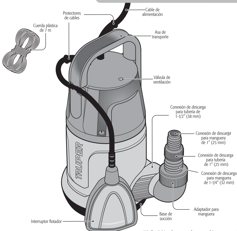
(A) Posición de apagado para el interruptor flotador
