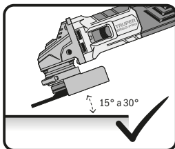
forma correcta de operar la esmeriladora para procesos de desbaste
