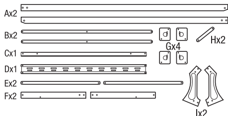
Partes de la base del calentador solar
