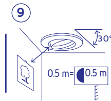
Distancia mínima de montaje
