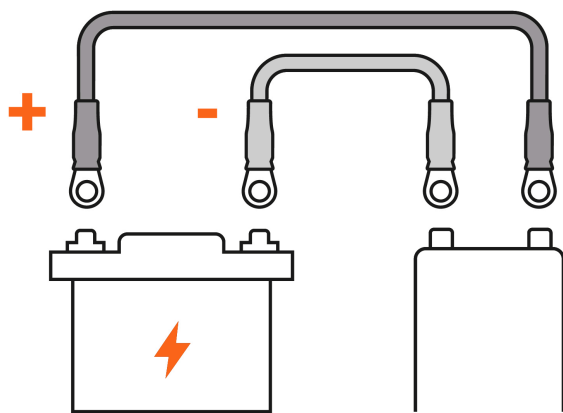
Conexión de batería a inversor
