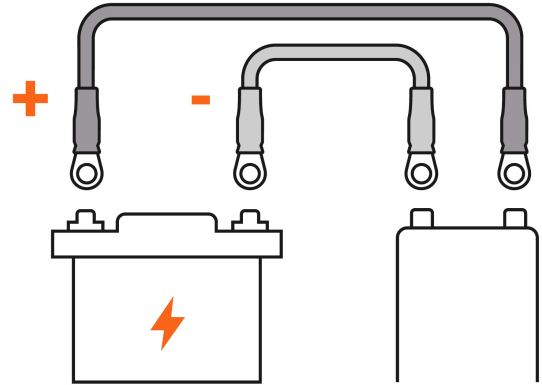
Conexión de batería a inversor
