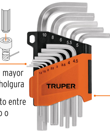
Punta recta con chaflán
