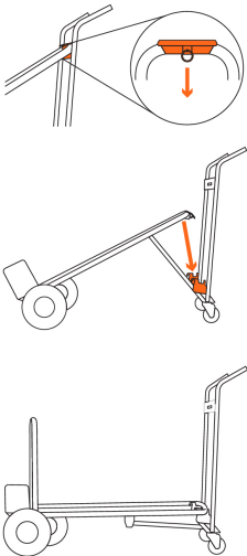
CONVERSIÓN DE ASISTIDO A 4 RUEDAS
