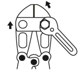
Alinee las cuchillas girando los tornillos hacia adentro
