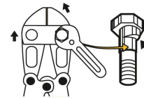
Una vez alineadas las cuchillas apriete las tuercas
