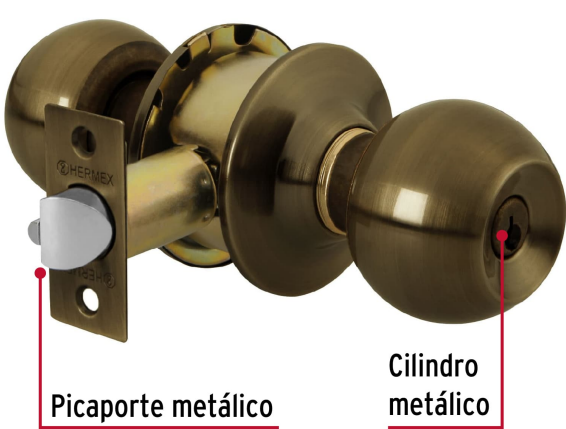
Mecanismo cilíndrico
