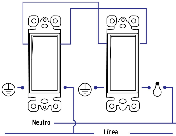
Diagrama de conexión
