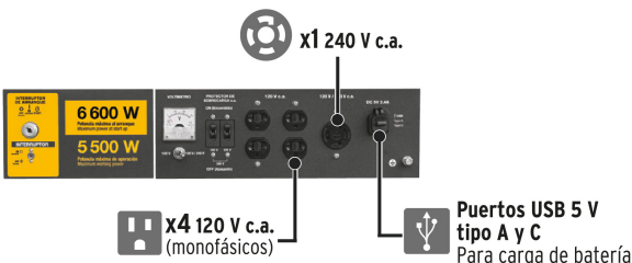
Páneles de control GEN-55P
