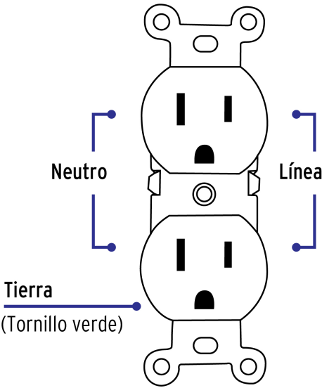
Diagrama de conexión
