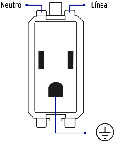
Diagrama de conexión
