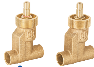
Conexiones roscables 1/2" - 14 NPT
