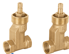
Conexiones roscables 1/2" - 14 NPT
