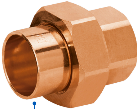
Conexiones soldables de 3/4" (19 mm)
