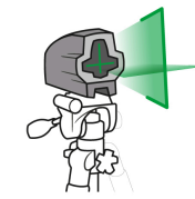
Niveles láser
