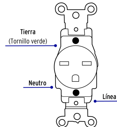
Diagrama de conexión
