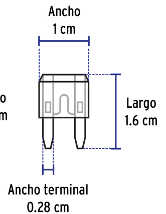
Fusible mini
