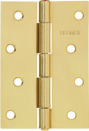
Perno remachado con cabeza media bola
