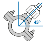
Fijar abrazadera a 45°
