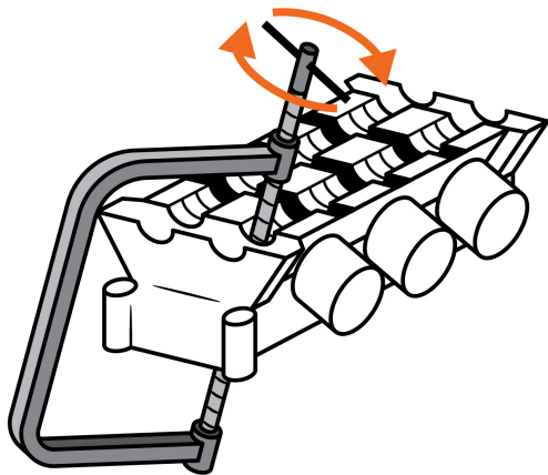
Para comprimir resortes de suspensión tipo McPherson®
