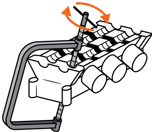
Para comprimir resortes de suspensión tipo McPherson®
