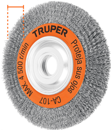
Diámetro 8" (200 mm)
