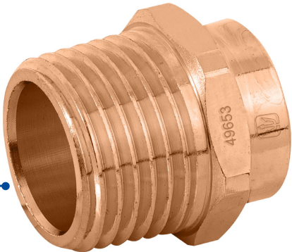
Conexión roscable de 1/2" NPT
