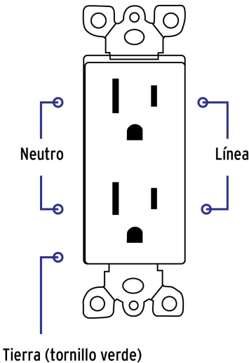
Diagrama de conexión
