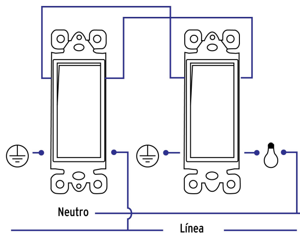
Diagrama de conexión
