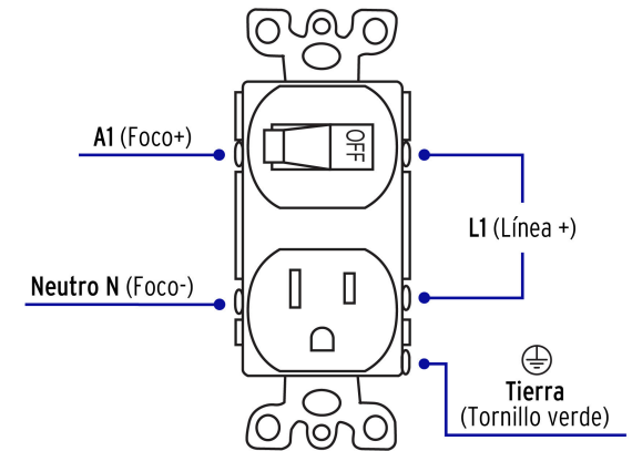
Diagrama de conexión
