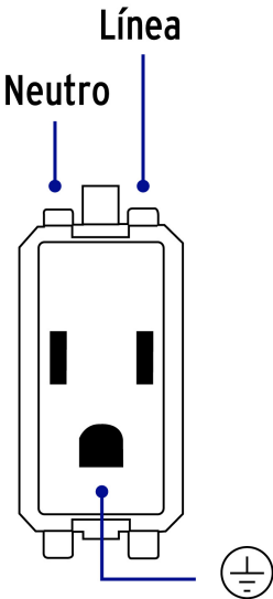
Diagrama de conexión
